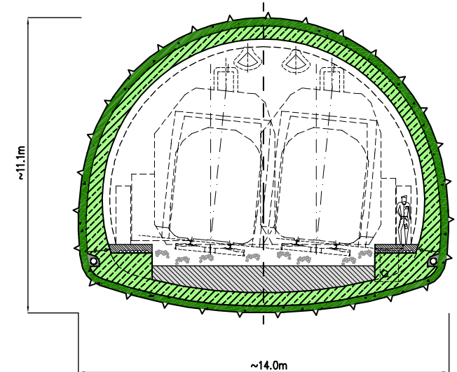
Querschnitt mit Sohlgewölbe
