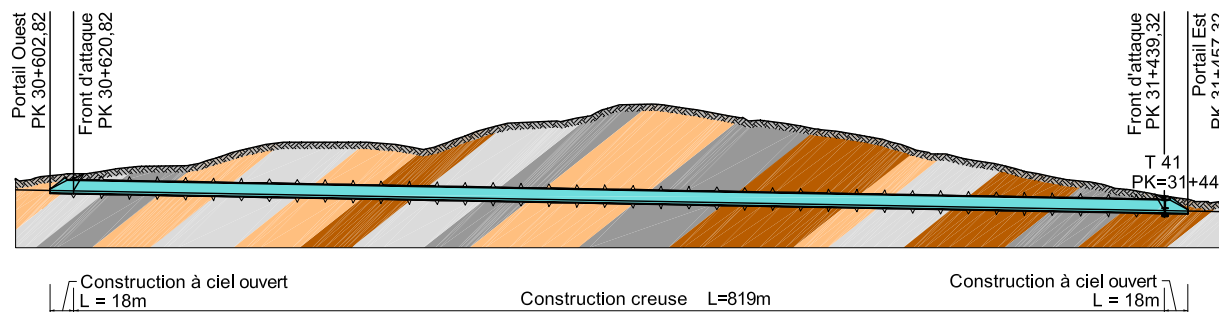
Längsschnitt mit Geologie (Wechsellagerung aus Sand-, Schluff-, Ton- und Mergelgesteinen)
